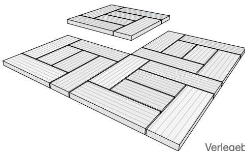
Verlegebild: Standardverband
