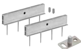
Holz Adapter Set, direkte Verschraubung auf Türblatt, Tragkraft 80 kg
